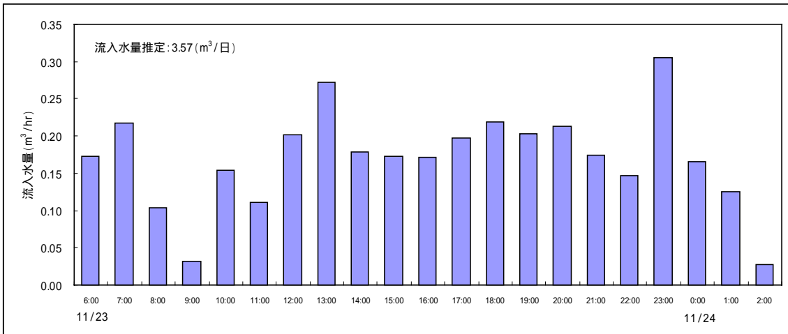
図5-1 流入水量の日間変化
