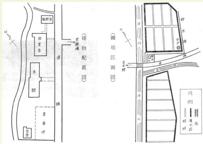
敷地の配置図
