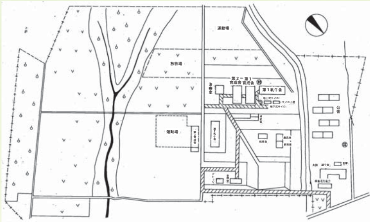
敷地の配置図
