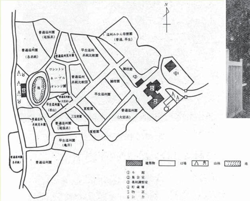
敷地の配置図
