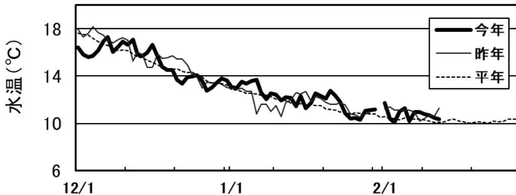
図2 西風成分の平年偏差
