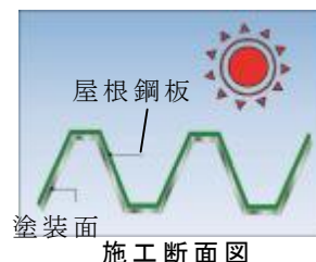
施工断面図
