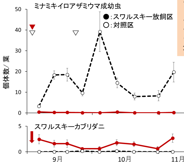
図. 施設キュウリにおけるスワルスキーカブリダニの放飼によるミナミキイロアザミウマの防除効果(2017年、富田林市) エラーバーはSE
